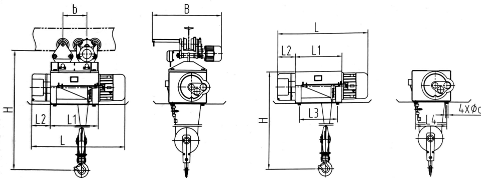
YH II 2-5吨 (H=9-20米)
