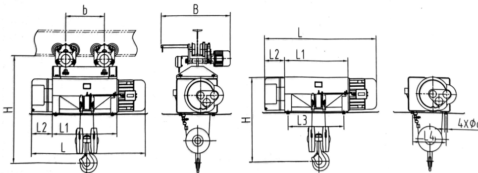
YH II 固定式10吨 (H=9-20米)
